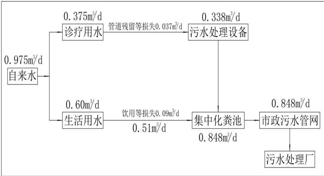
图 4 项目水平衡图
